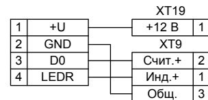
«Сигнал-ВК6»
