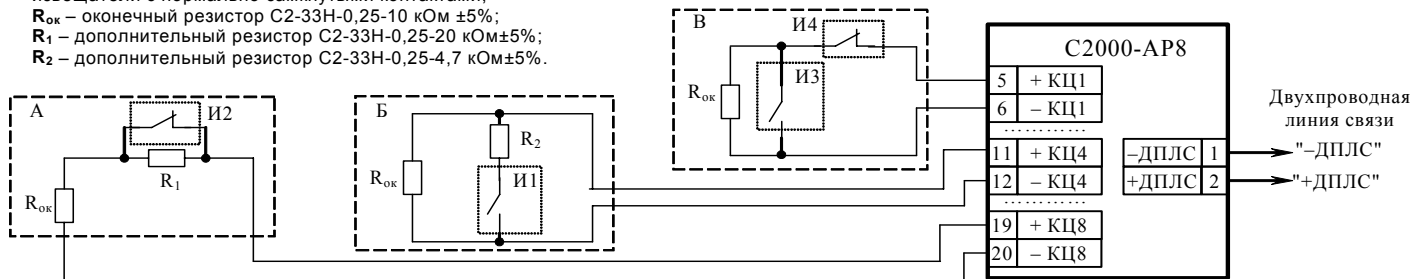
Рисунок 1 Схема соединений
