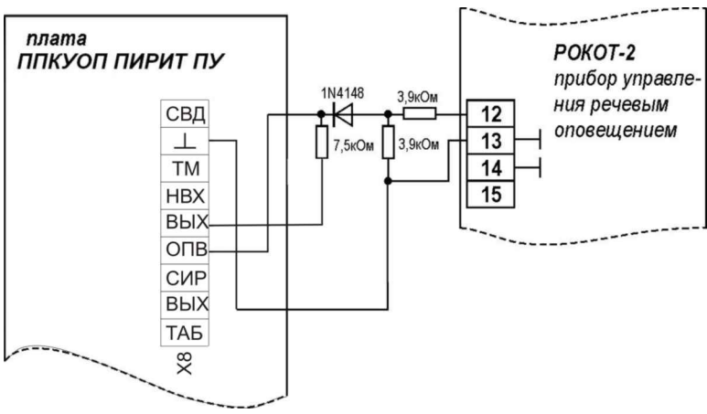
Рис. 8 Подключение прибора речевого оповещения «РОКОТ-2»
