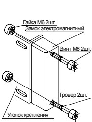
Рис. 1. Вариант крепления электромагнитного замка к раме двери.
