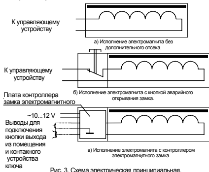
Рис. 3. Схема электрическая принципиальная.
