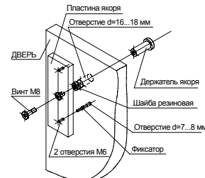
Рис. 2. Монтаж пластины якоря.
