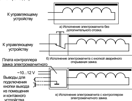
Рис. 3. Схема электрическая принципиальная.
