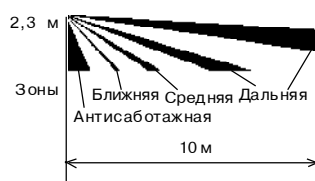
Рис. 5 Диаграмма зон обнаружения
